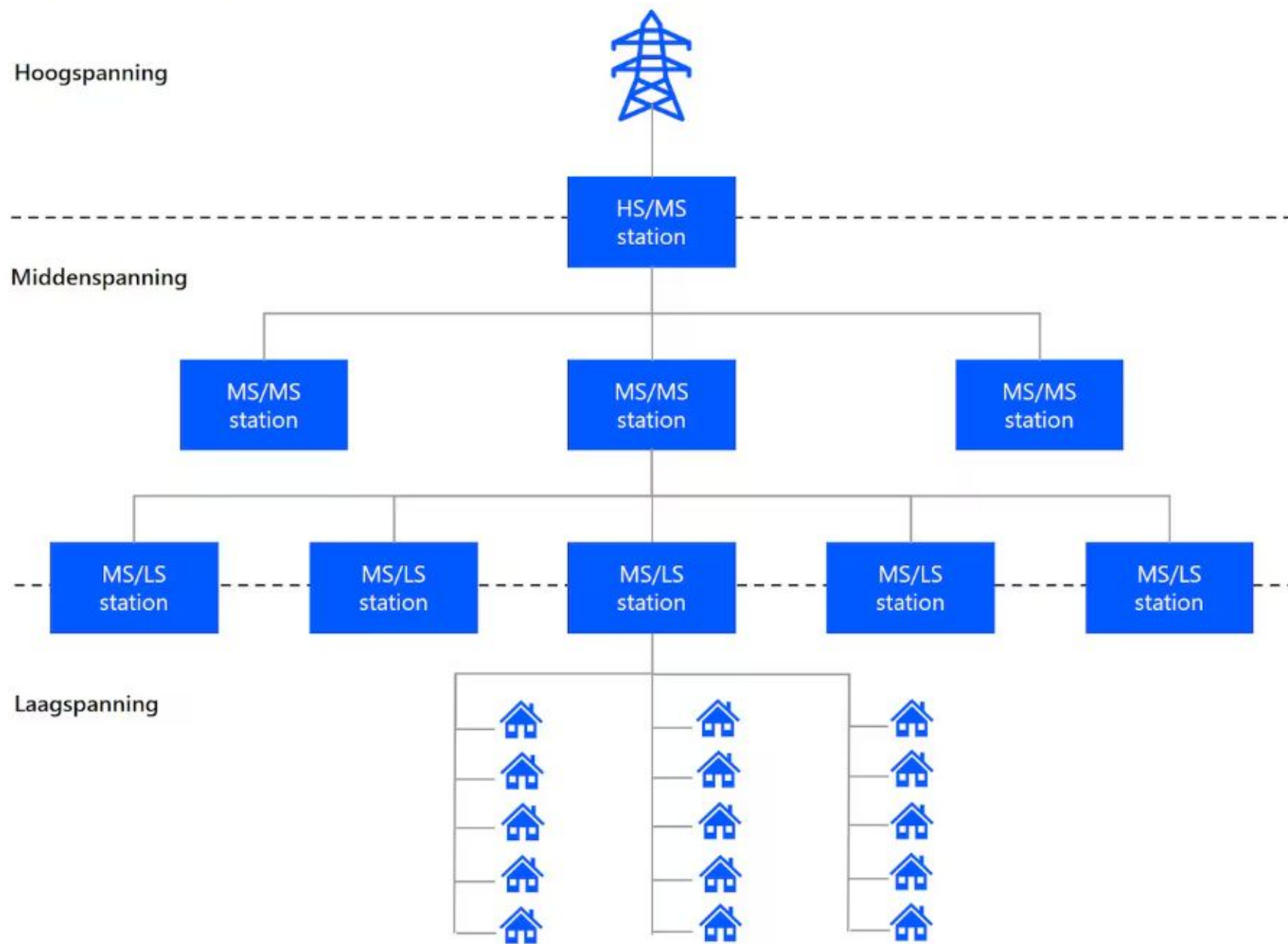
Figuur 1: Versimpeld schematisch overzicht van elektriciteitsinfrastructuur
