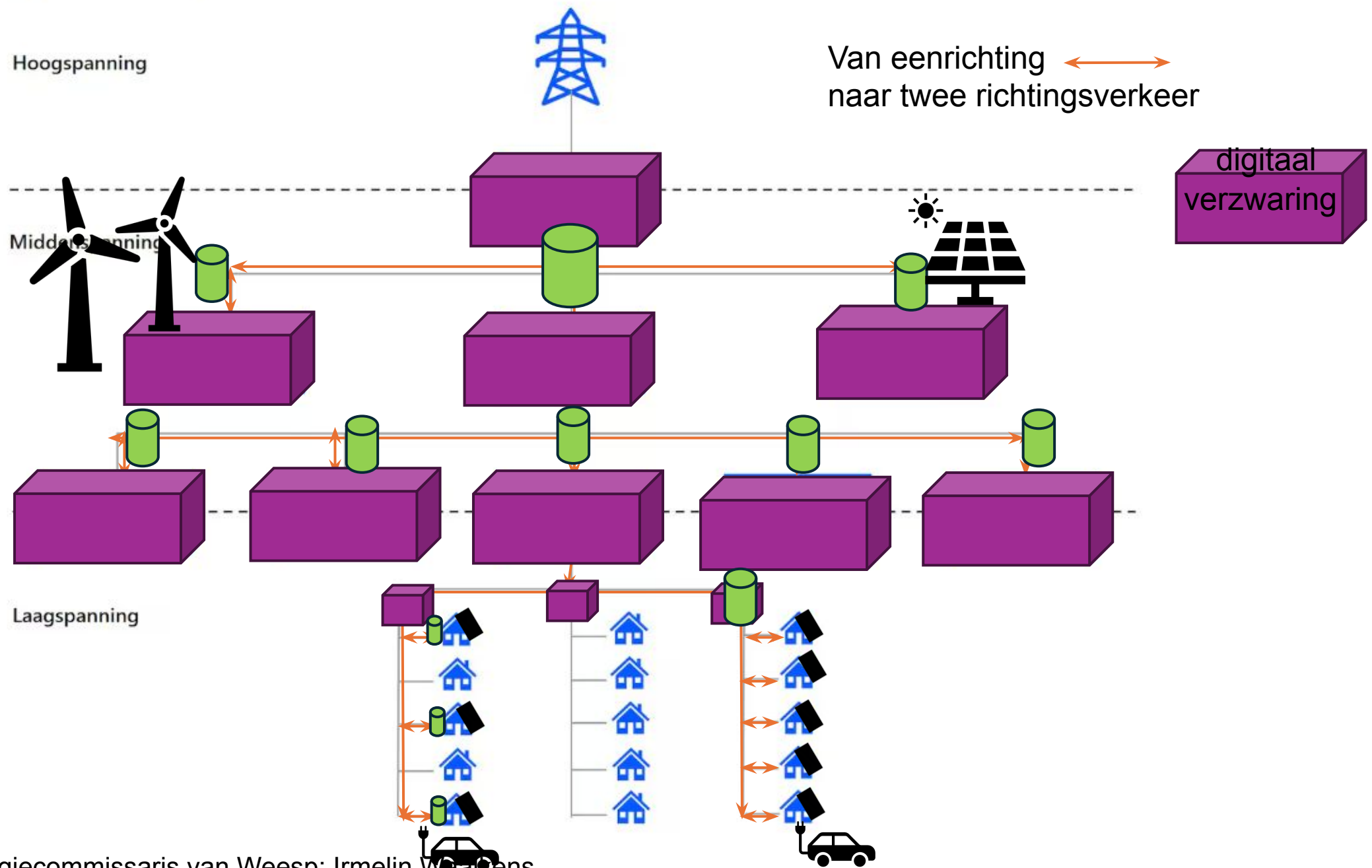
Figuur 1: Versimpeld schematisch overzicht van elektriciteitsinfrastructuur
